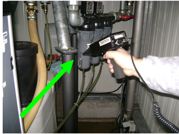
En sortie de compresseur : 1 ère fuite sur le réseau 6-8 Bars
