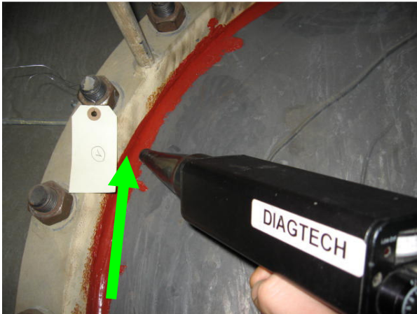
Cuve en dépression / problème de vide
