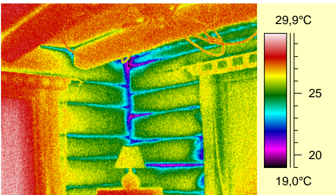
Maison à structure bois
