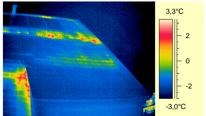
Maison individuelle à structure traditionnelle.
